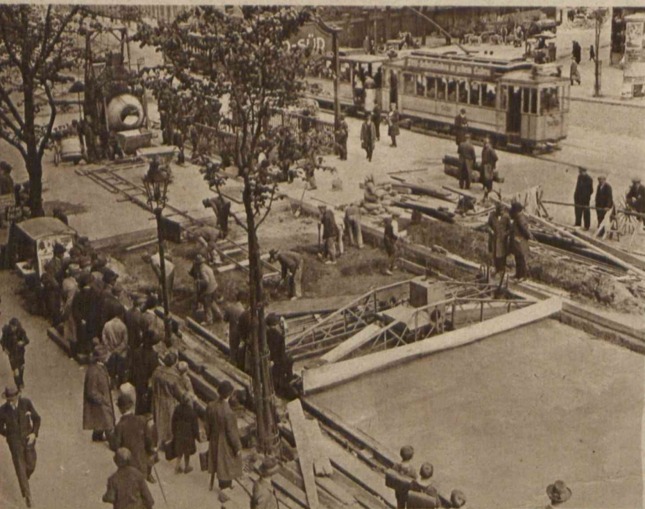
Maszyna do budowy ulic, która w ciągu 4 dni buduje 1 km. drogi. Na szerokości 9 m. posuwa się maszyna, ugniatając rozsypany poprzednio beton. Po kilku godzinach przestrzeń ugnieciona gotowa jest do użytku. Maszynę obsługują tylko 2 robotnicy.
