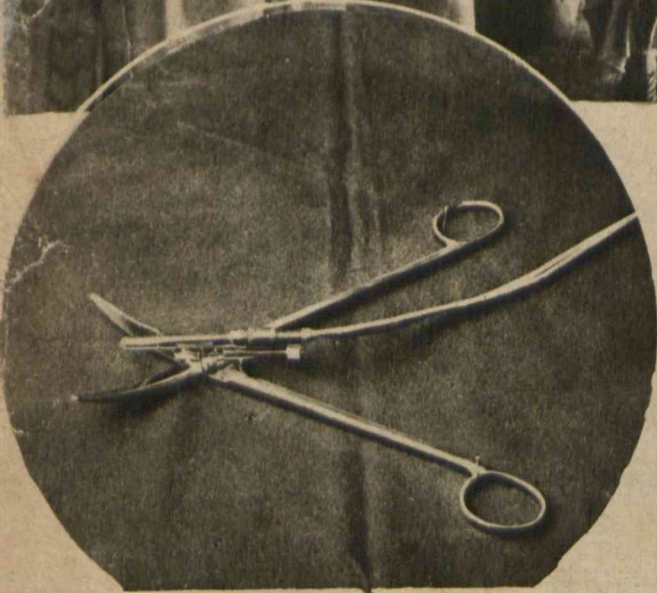
Wynalazek lekarza-berlińskiego Haelbera: świecące nożyce chirurgiczne, ułatwiające chirurgowi pracę przy głębokich operacjach wewnętrznych. Na końcu instrumentu znajduje się lampka elektryczna, którą można wygotować i dezynfekować.
