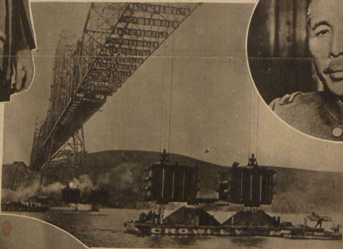
U dołu: Z budowy olbrzymiego mostu w Carquinez Straits (St. Zjedn.). Potężne łuki mostu dla przeciwwagi obciążone są od dołu wagonami z piaskiem, które się w odpowiednim momencie opróżnia.
