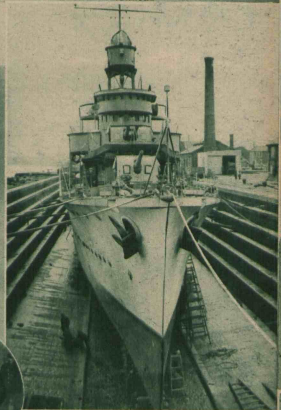
Nowy kontrtorpedowiec polski „Grom” w porcie Southamptona po ostatecznym wykończeniu
