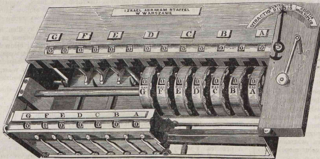
Machina rachunkowa I. A. Staffla w Warszawie.
