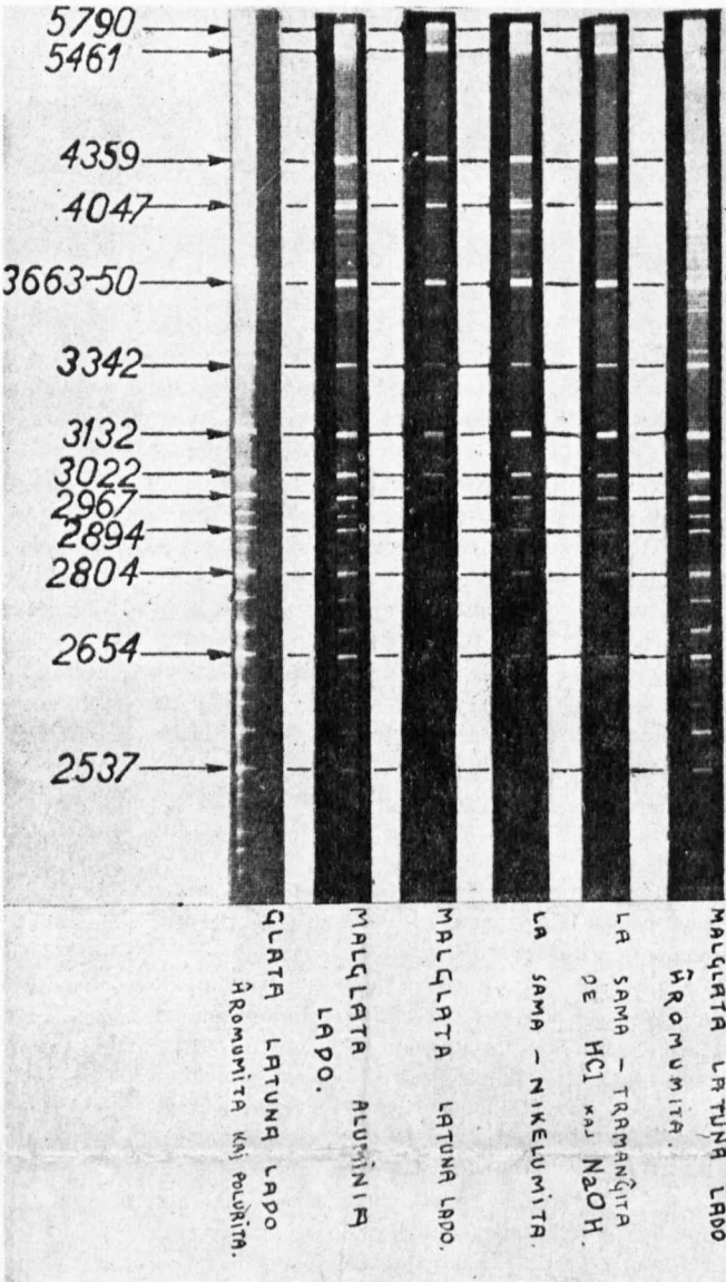
Ilustraĵo 4 Spektro de lumo reflektigata kaj dispersigata de diversaj metaloj
