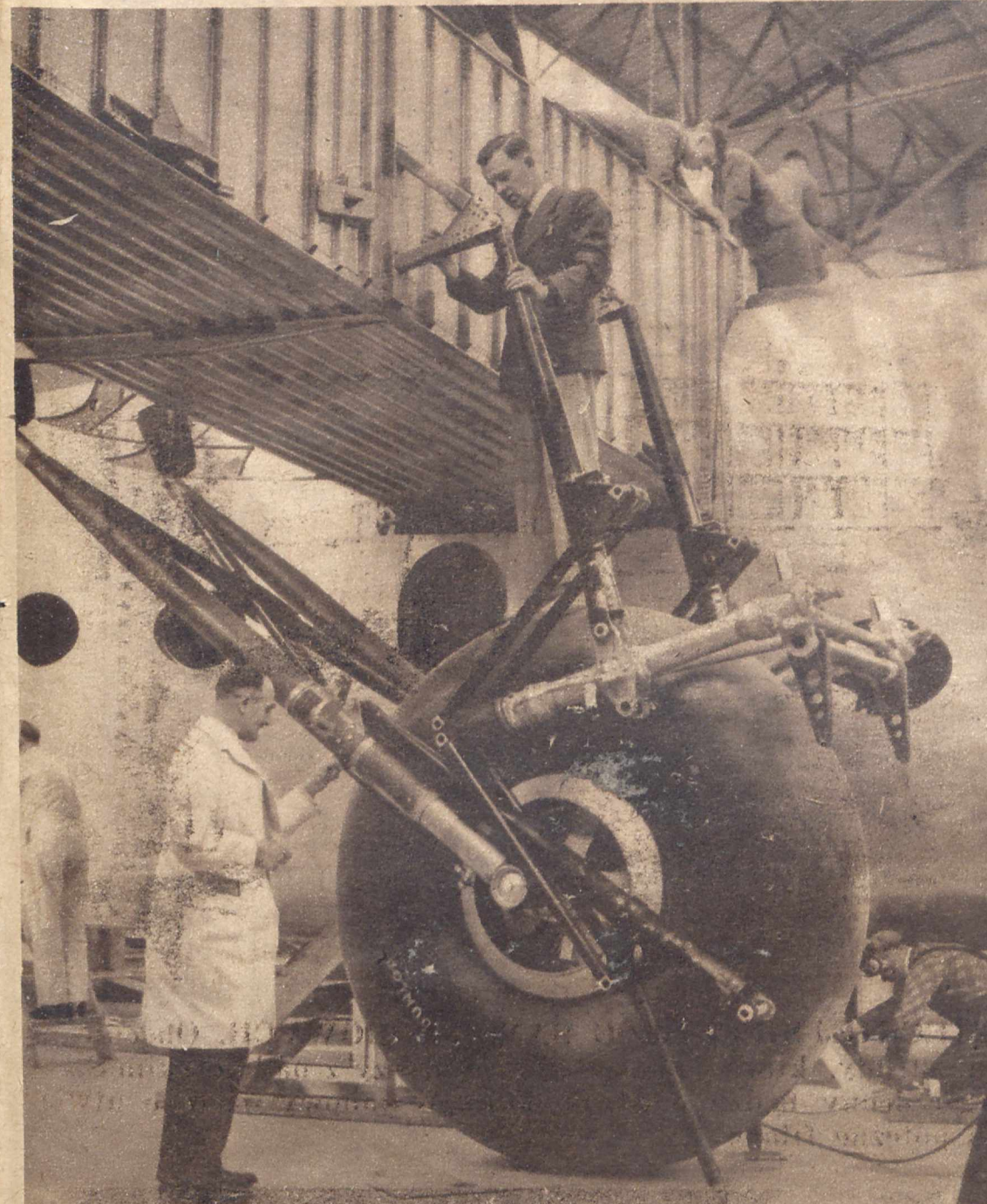
BUDOWA OLBRYZMICH SAMOLOTÓW PASAŻERSKICH. Światowej sławy wielka fabryka angielska Armstrong Whitworth w Southampton, której nazwa pojawia się obecnie bardzo często w sprawozdaniach o zakrojonej na wielką skalę angielskiej akcji dobrobroniowej, pracuje równocześnie nad budową gigantycznych samolotów pasażerskich dla komunikacji pomiędzy Anglią a koloniami.
