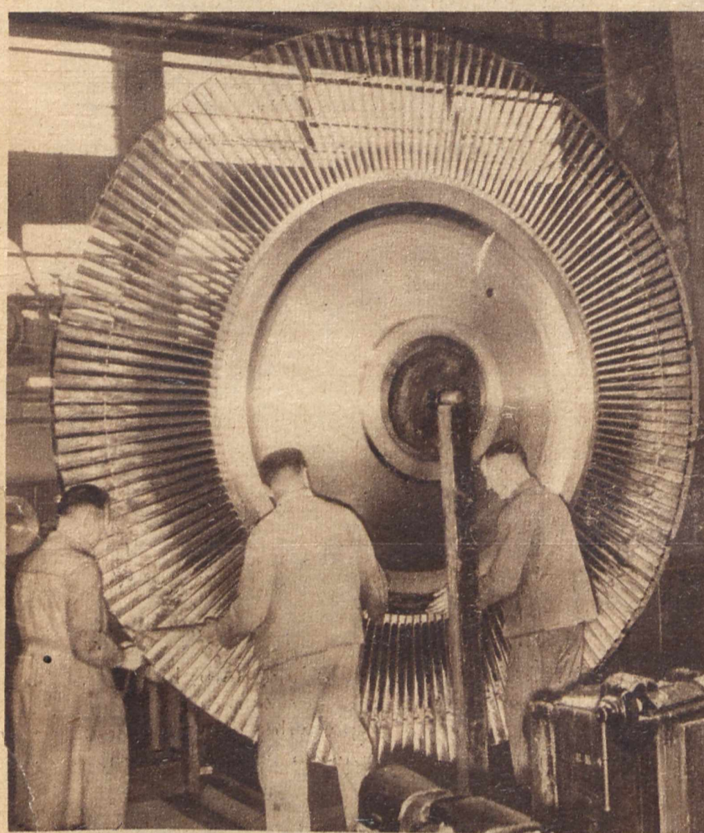
OLBRZYMLIA TURBINA PAROWA. Ugoda niemiecko-japońska, niedawno zawarta, ma na celu nietylko współdziałanie polityczne, ale również — a może przede wszystkim — współdziałanie w dziedzinie przemysłu i handlu. Doskonale na tem wychodzą niemieckie fabryki maszyn. Tak np. w jednej z nich Japonia zamówiła olbrzymią turbinę parową o sile 60.000 koni parowych.
