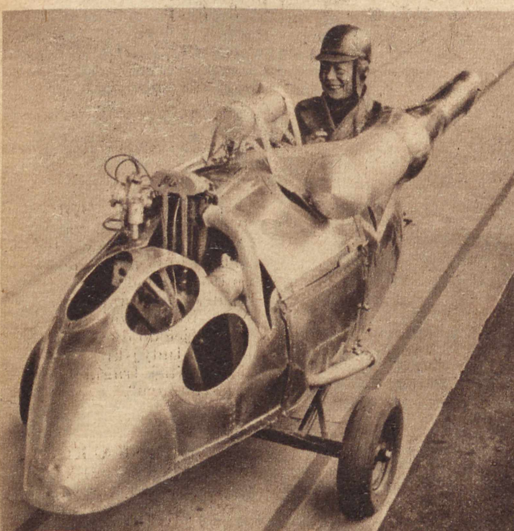
ORYGINALNY MODEL SAMOCHODU. Francuski inżynier Lisois jest twórcą tego niezwykłego typu samochodu wyścigowego, który popędzany sprężonym powietrzem może rozwinać szybkość do 200 km. na godz. Wóz ten, nazwany rakieta posiada tylko trzy koła.
