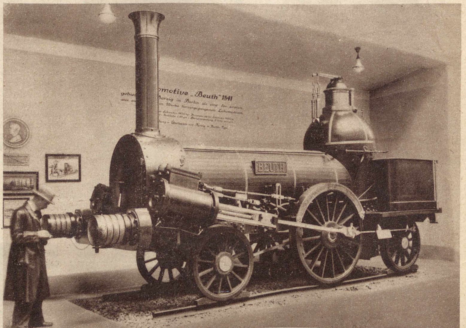
STO LAT KOLEI! Oto model lokomotywy „Beuth” z roku 1841. Była to jedna z pierwszych maszyn, wyprodukowana przez fabrykę Borsig w Niemczech. Obecnie przeszła do muzeum kolejowego.
