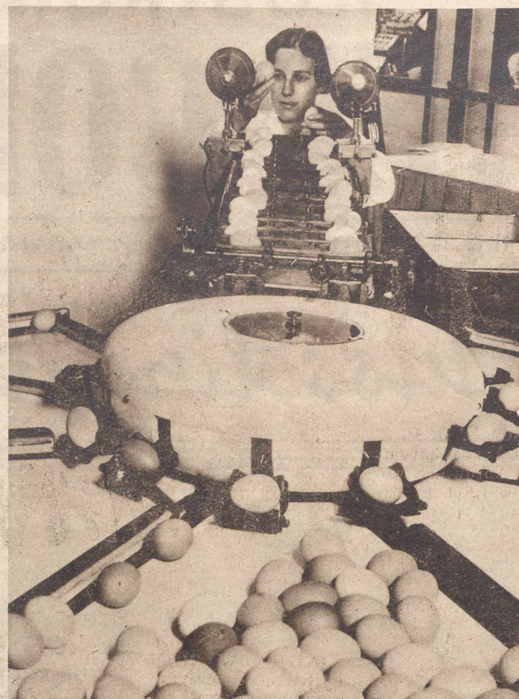
AUTOMATYCZNE SORTOWANIE JAJ. Na wystawie kolonialnej w Londynie zademonstrowano maszynę do sortowania jaj, które po prześwietleniu odkłada aparat stosownie do wagi.
