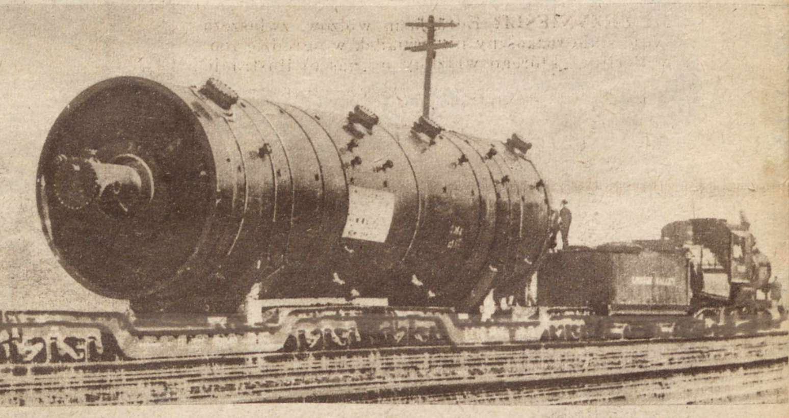
OLBRZYMI ZBIORNIK NAFTY. W celu przetransportowania jednego z największych zbiorników nafty musiało Towarzystwo Standard Oil Co. w Jersey City zbudować specjalną platformę. Zbiornik odbył podróż koleją, a następnie przez morze holowany przez parowiec na przestrzeni 2.000 km. Ciężar przedstawionego na naszej ilustracji zbiornika wynosi 230.000 kg.
