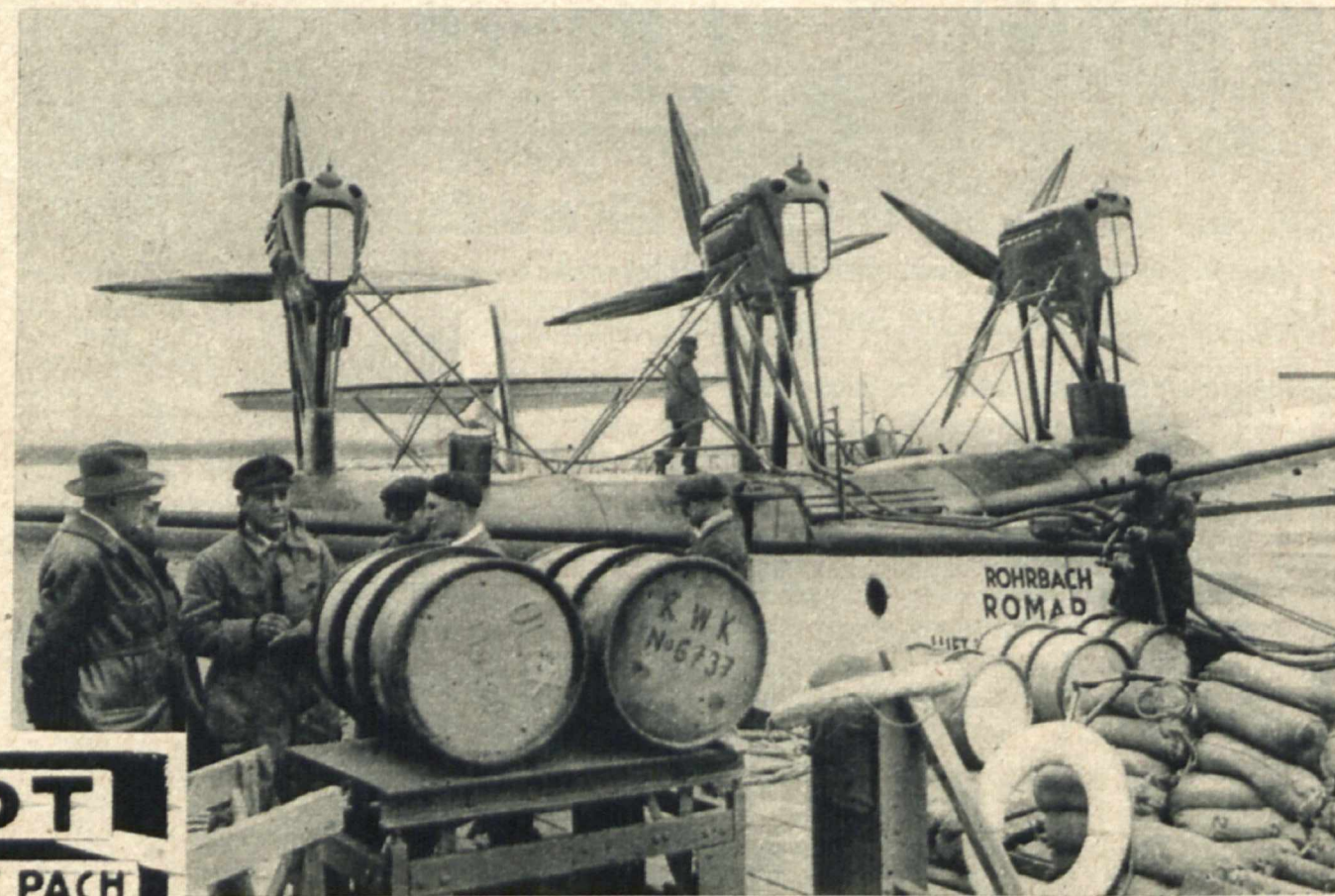
Nowy rekord w lotnictwie. Trójmotorowy olbrzymi aparat „Romar“, obciążony 6.450 kg., osiągnął w próbnym locie w okolicy Travemünde rekord wysokości, wznosząc się aż do 2.200 metrów. Dotychczasowy rekord wynosił przy 4.037 kg. ciężaru 2.000 m. wysokości.
